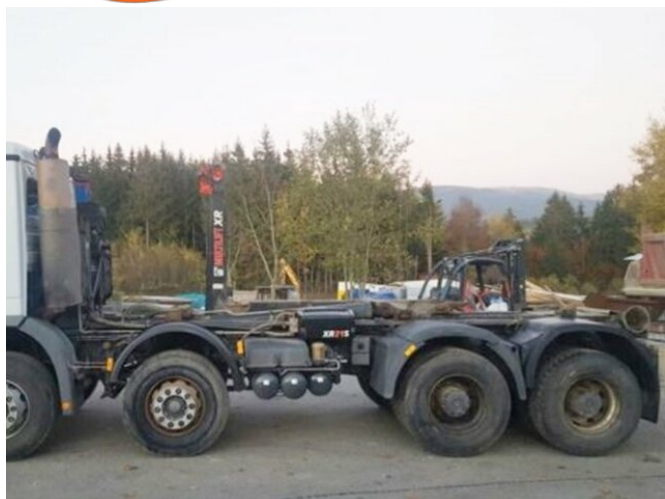
HIAB MULTILIFT XR21S59 Abrollanlage
