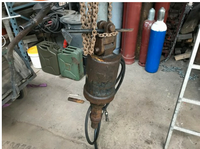
Kinshofer AS05 Antriebseinheit für Bohrschnecken
