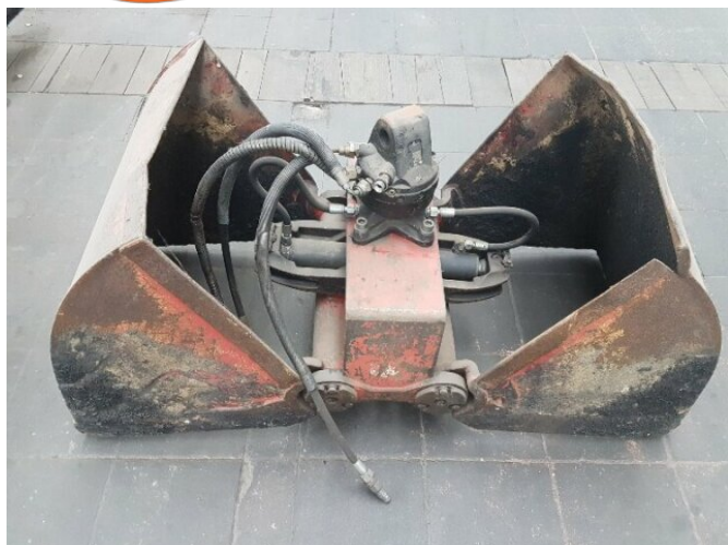
Kinshofer 2-Schalengreifer
