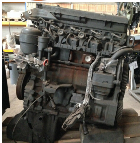
Mercedes-Benz OM 904
