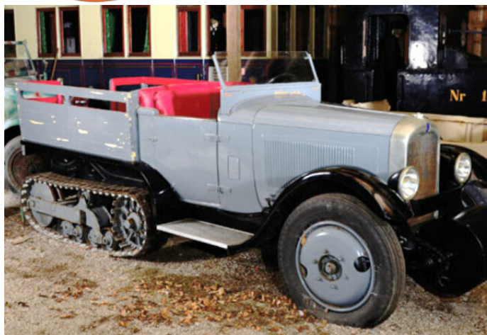
Citroen Citroen Kegresse Half-Track Kettenfahrzeug
