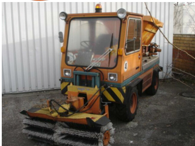
Bucher GT 1200B 4x4
